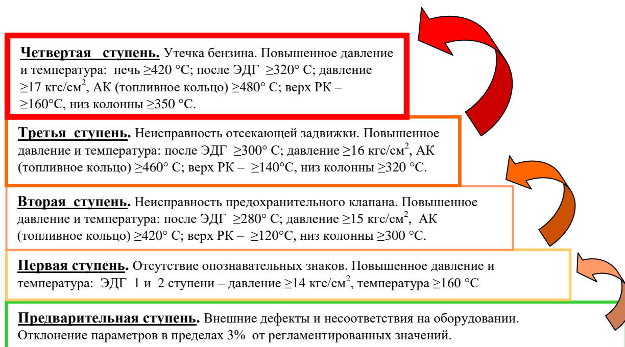
Рисунок 4. «Лестница принуждения» для установки АВТ-6
