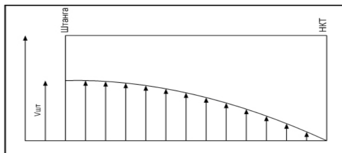
Рисунок 4. Профиль скорости жидкости в кольцевом пространстве НКТ при D_{нкт} = D_{син}
