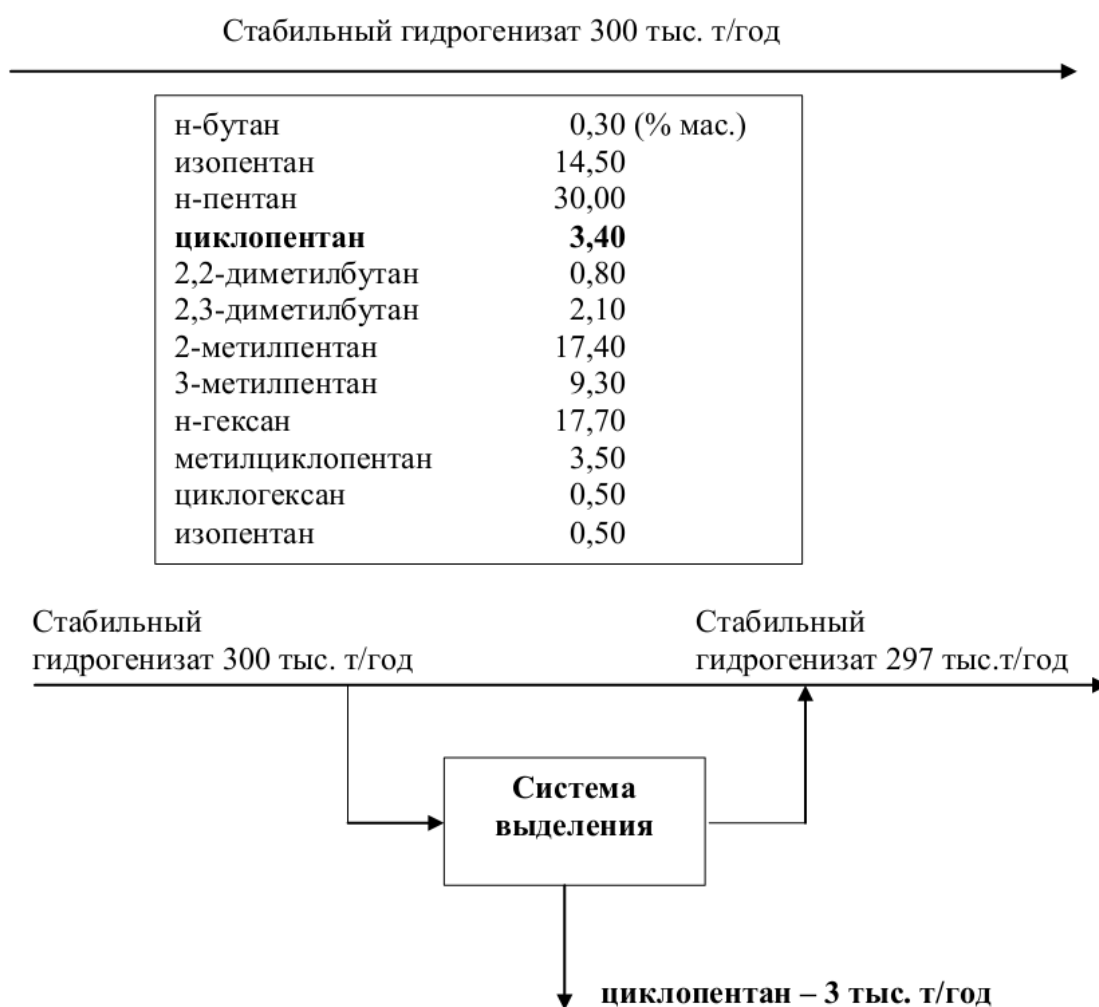
Рис. 7. Встраиваемая технология выделения циклопентана
