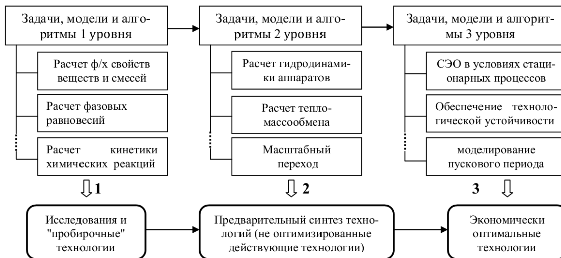
Рис. 1. Уровни моделирования при создании новых и модернизации действующих производств
